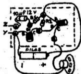
EL CIRCUITO ARMADO CON SEIS TORNILLITOS
