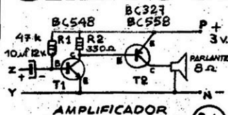
AMPLIFICADOR
