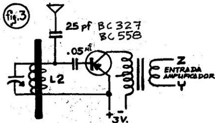
La alimentación de 3 v. se toma de las mismas pilas del amplificador
